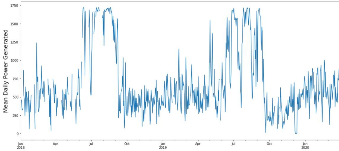
Görsel 5. Örnek rüzgâr çiftliğinin güç çıkışı.
