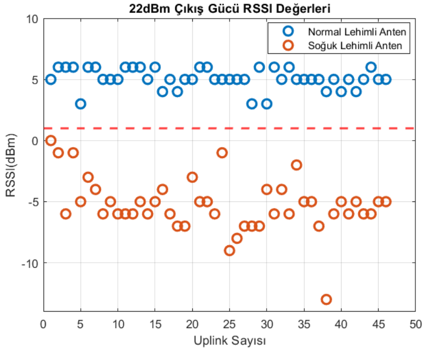
Görsel 11. 22dBm çıkış gücü için normal lehimli ve soğuk lehimli anten kullanılarak yapılan test sonuçları
