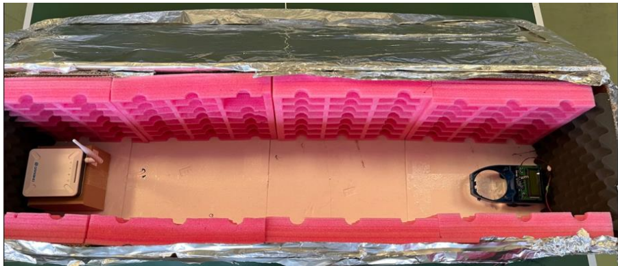
Görsel 9. Test ortamı.
