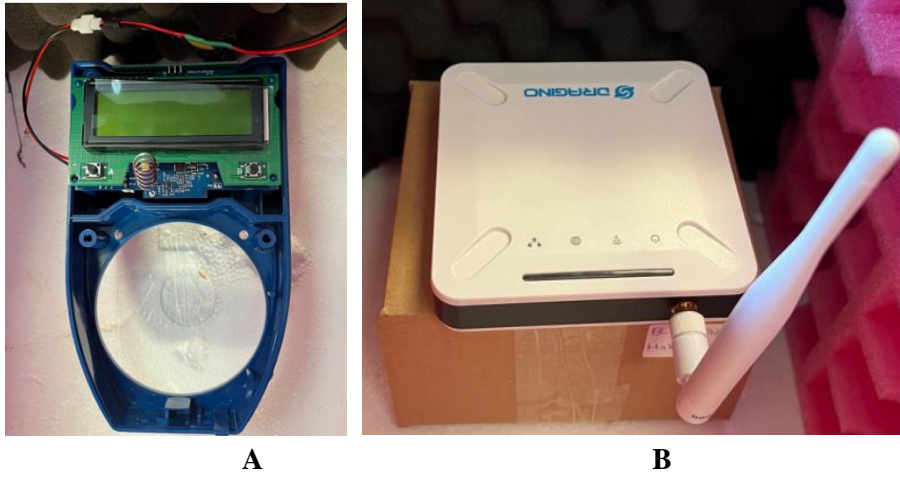
Görsel 6. A- Transmitter: Baylan AK-311 LoRa su sayacı elektronik devresi, B- Gateway Dragino indoor gateway(LPS8).
