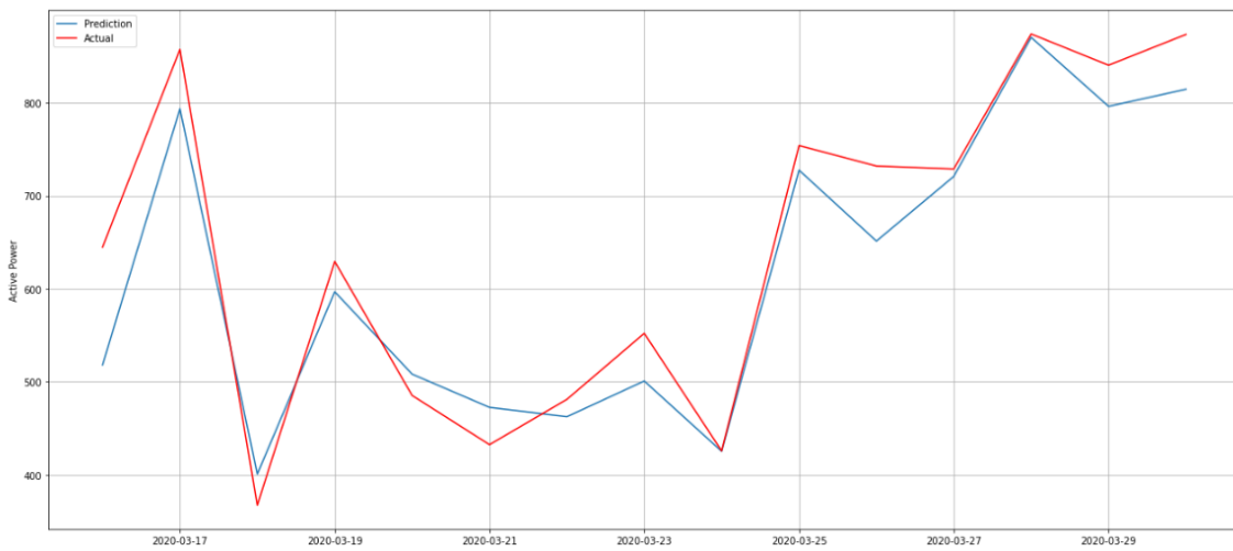
Görsel 7. Rüzgar gücü tahmininin ikinci sonucu.
