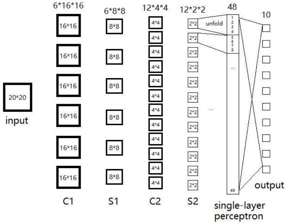
Görsel 4. ESA yapısı.
