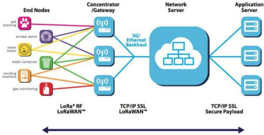
Görsel 1. LoRa ağ yapısı.
