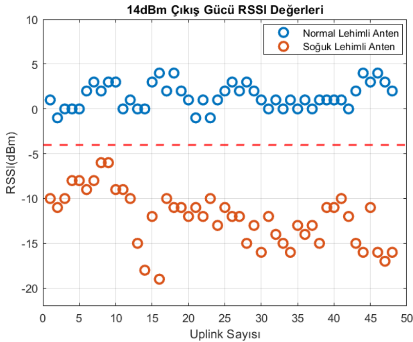
Görsel 10. 14dBm çıkış gücü için normal lehimli ve soğuk lehimli anten kullanılarak yapılan test sonuçları.
