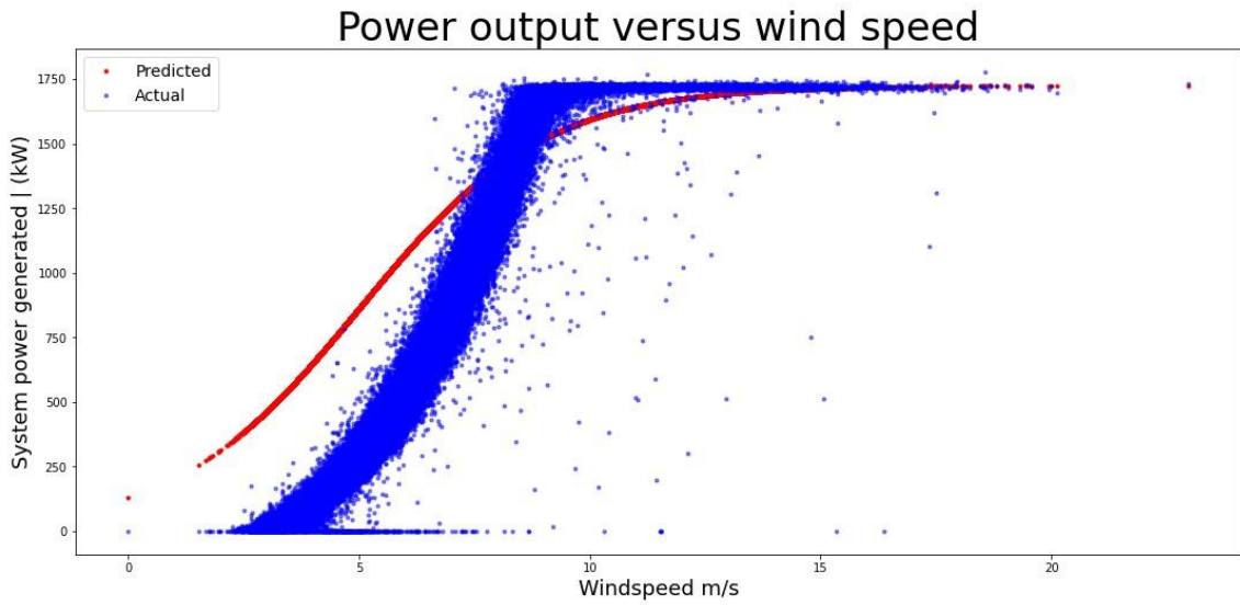
Görsel 5. Rüzgâr gücü tahmini
