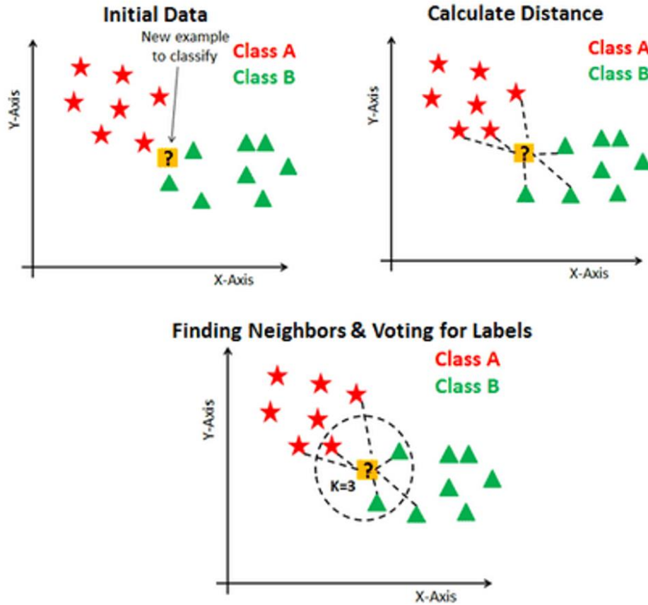
Görsel 1. KNN regresyon modeli
