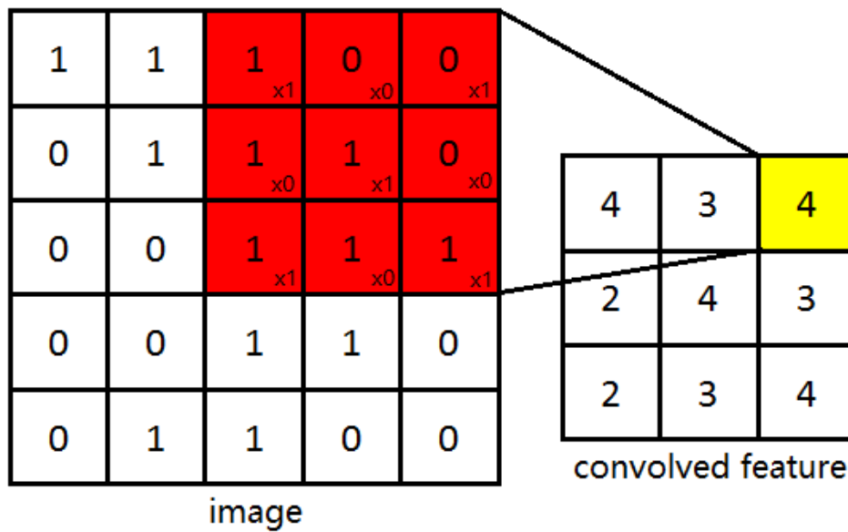
Görsel 2. Konvolüsyon süreci.
