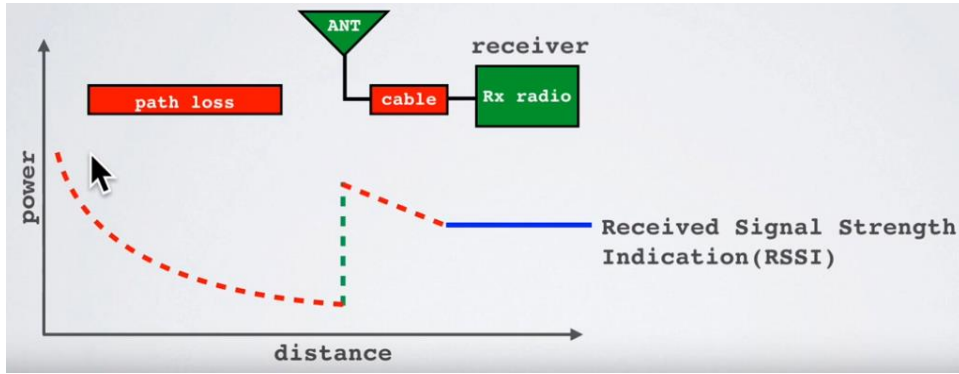
Görsel 2. RSSI kavramının açıklanması [8]
