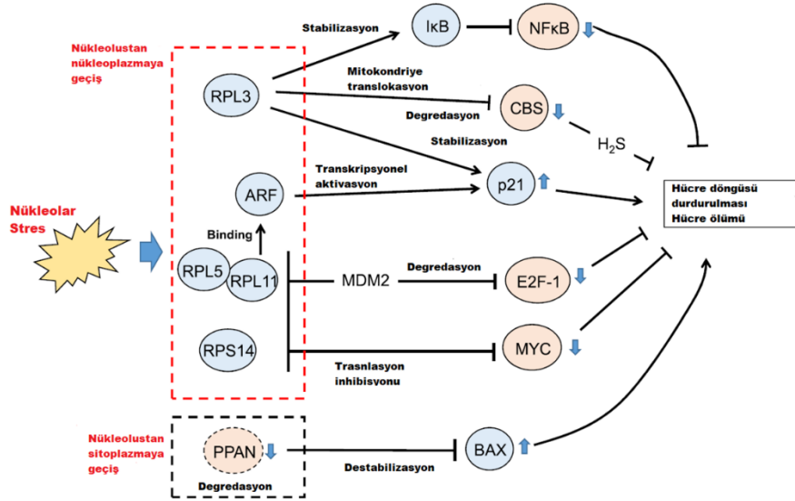
Şekil.3 p53'ten bağımsız nükleolar stres yanıt yolları (3).
